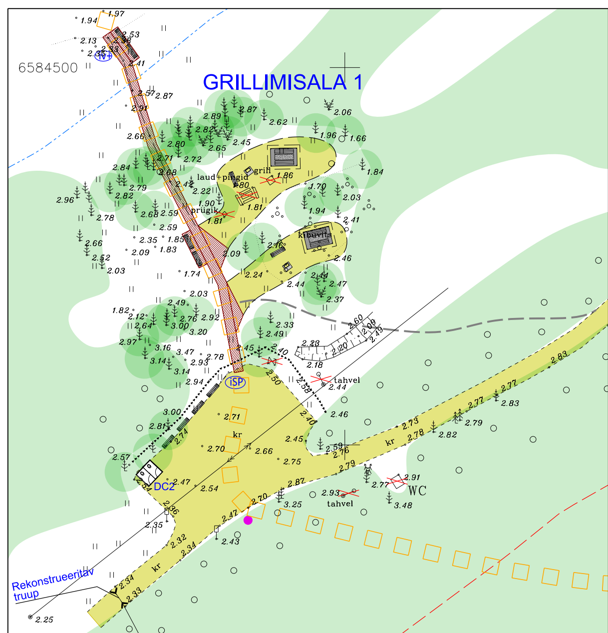
GRILLIMISALA 1 M 1:500
